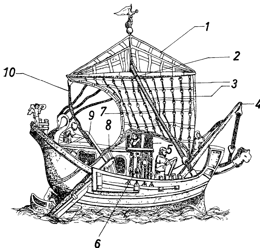
1: Amantillo.—2: Estay.—3: Brioles.—4: Botalón.—5: Obenques.—6: Bigota. 7. Relinga.—8: Escota.—9: Caña.—10: Braza.
