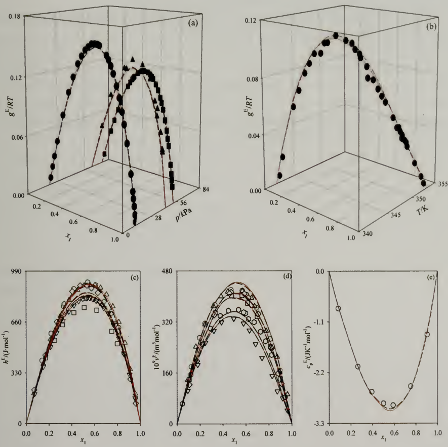
Figura A-3. Representación de los valores experimentales de diferentes cantidades termodinámicas y las curvas de correlación obtenidas mediante la versión D, con los parámetros k_g, k_h, k_v y k_c determinados en el proceso de ajuste (—), y la versión F del modelo con los parámetros k_g, k_h, k_v y k_c como función de p y T según las expresiones (A.5), (A.7), (A.10) (---) frente a la concentración del sistema binario x_1 Benceno+ x_2 Hexano (12) de la Tabla 2 y 3. (a) Función de energía de Gibbs de exceso del ELV isotérmico a T = 298.15 K (■), T = 328.15 K (▲) y T = 333.15 K (●). (b) Función de energía de Gibbs de exceso del ELV isobárico a p = 101.32 kPa (●). (c) Entalpía de exceso a T = 293.15 K (○), T = 298.15 K (△), T = 313.95 K (□), T = 318.15 K (◇) y T = 323.15 K (▽). (d) Volumen de exceso a T = 288.15 K (○), T = 298.15 K (△), T = 303.15 K (□), T = 308.15 K (◇), T = 318.15 K (▽) y T = 323.15 K (●). (e) Capacidad térmica de exceso a T = 298.15 K (○).
