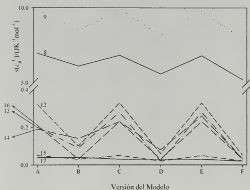
Figura 5. Desviaciones estándar, s(y) , con las diferentes versiones del modelo de la Tabla 1, aplicados en la correlación de los sistemas de la literatura. Los números indican la asignación del sistema según la Tabla 3, y considerando el parámetro k_{ij}(p,T) .
