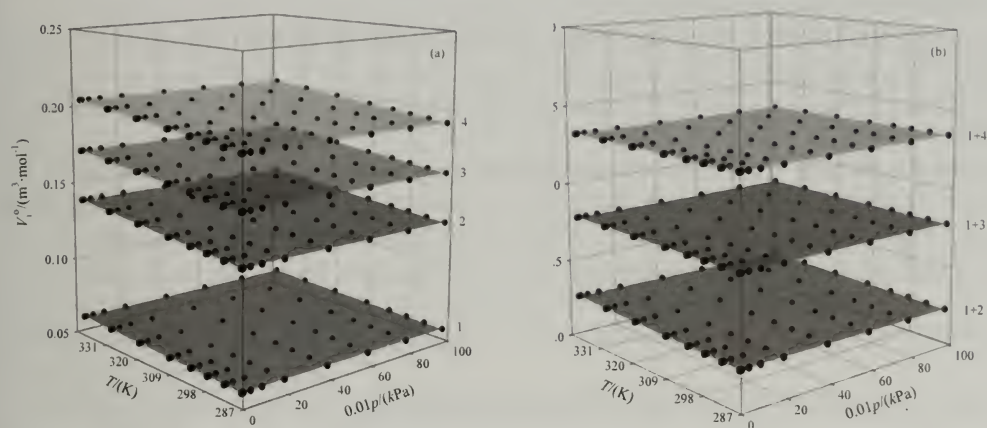
Figura A-1.- (a) Representación de la variación de los volúmenes molares V_m^o , de compuestos puros (1:etanol, 2:hexano, 3:octano, 4:decano) con la presión y la temperatura. (b), Variación del parámetro k_{ij} de las mezclas binarias indicadas con los compuestos anteriores, con la presión y la temperatura.
