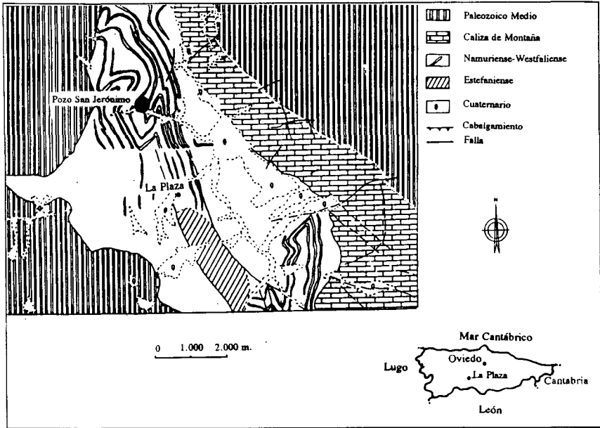
Figura 1.- Esquema geológico. Pozo San Jerónimo. Cuenca de Teverga.
