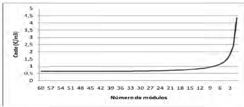
FIGURA 22: Evolución del coste del m 3 de agua desalada en función del número de módulos.
