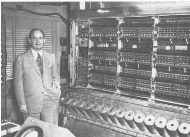
Von Neumann
