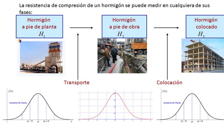
Figura 2. Uso de Distribuciones Estadísticas en Edificación.
