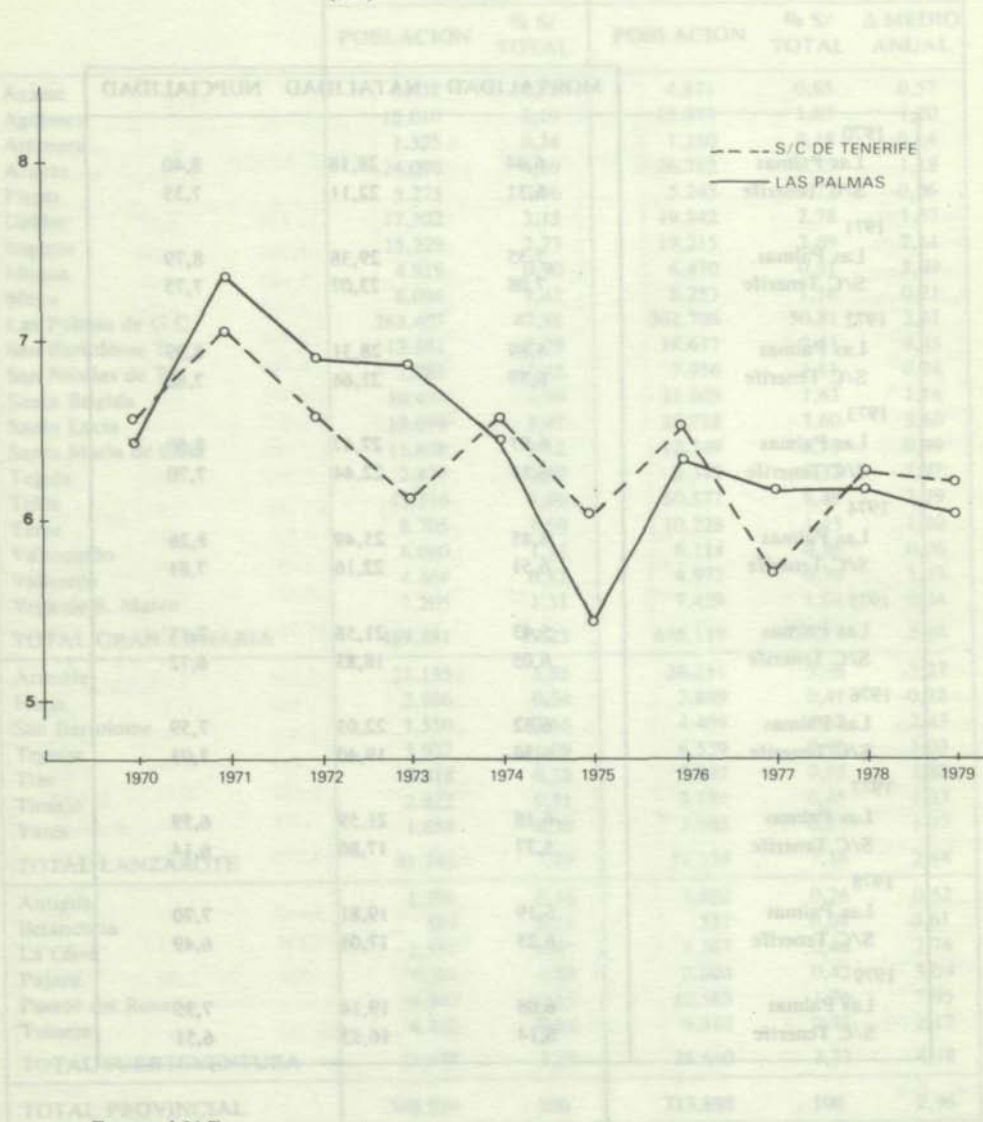
CUADRO I-1 POBLACION DE DESEMPEÑO EN LAS CANARIAS ORIENTALES A NIVEL MUNICIPAL (1970-1979) GRAFICO I-1 EVOLUCION DEL MOVIMIENTO NATURAL DE LA POBLACION (000) MORTALIDAD 1970-79
