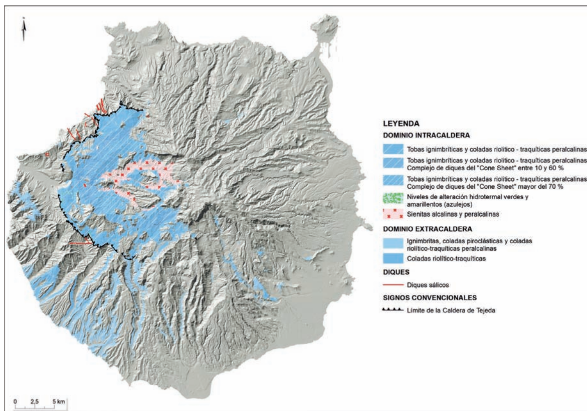
Fig. 9. Modelo de relieve sombreado de Gran Canaria con localización de las formaciones riolítico-traquíticas y los niveles de alteración hidrotermal (Azulejos). F: Mapa Geológico Digital Continuo de Canarias modificado por AT Hidrotecnia S.L, IGME-GRAFCAN, (2003).
