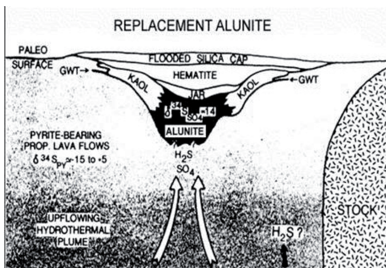
Fig. 8. Esquema del proceso hidrotermal de formación de alunita F: CUNNINGHAM y OTROS (1984).
