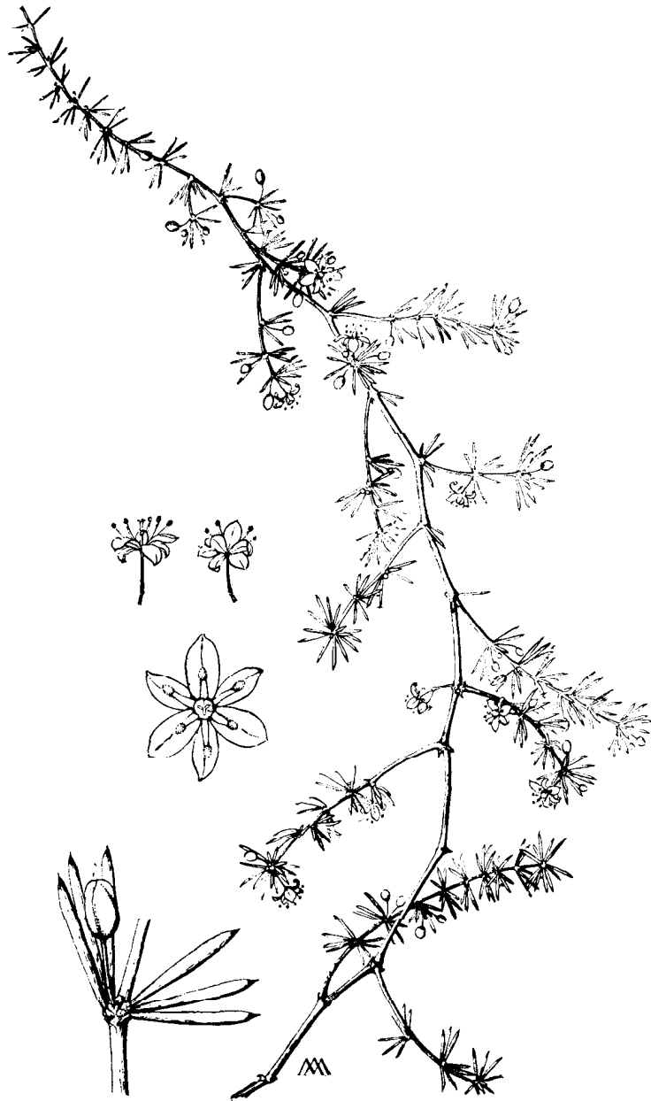
Asparagus nesiotes , rama florífera = \frac{1}{2} , dos flores = 1, flor diamétrica y detalle de filocladios = 2,5 — Dibujo por Mary Anne Kunkel.
