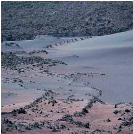
Rastro producido por las bolas de acreción en la ladera de Montaña Rajada.
