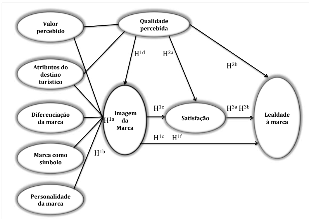
Figura 1. Modelo Conceptual
