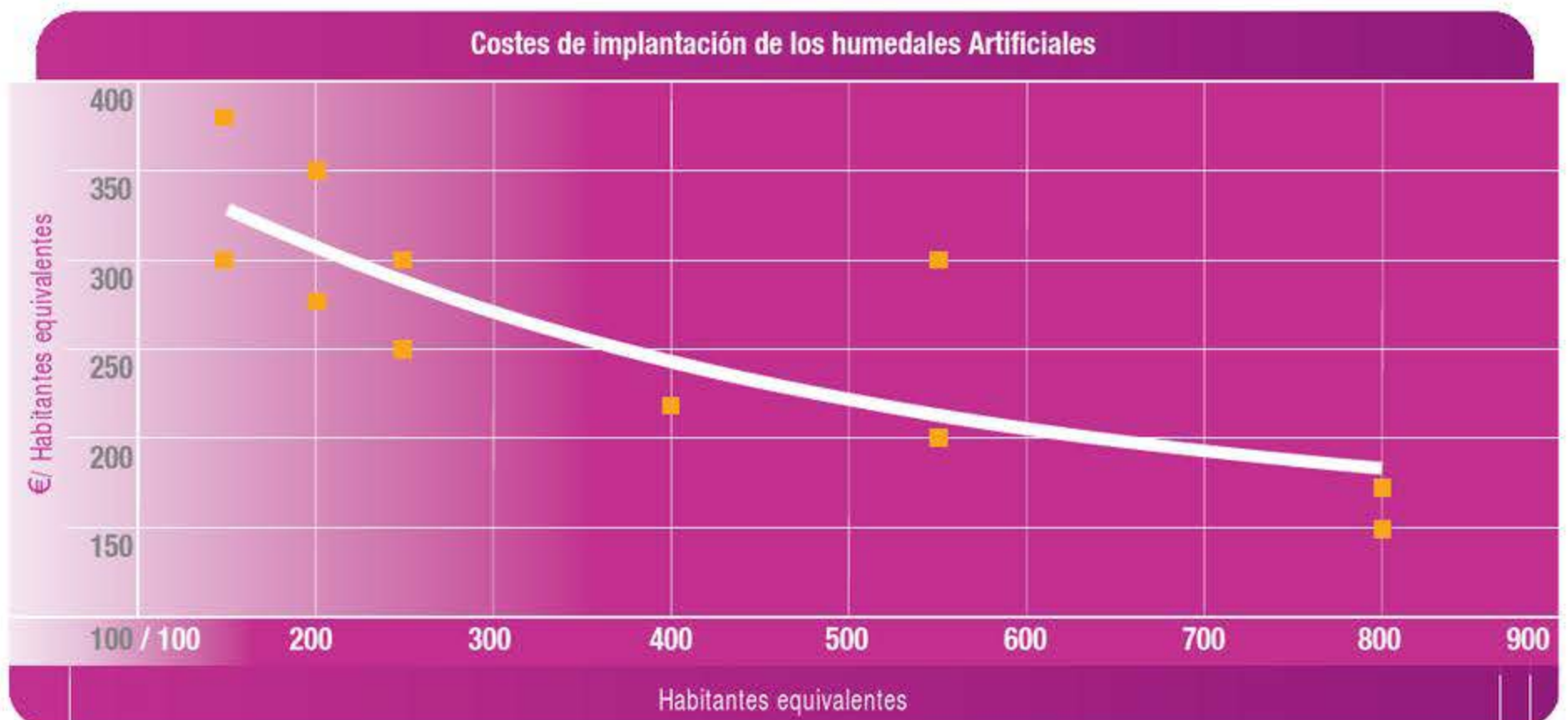
Figura 1. Costes de implantación de humedales artificiales
