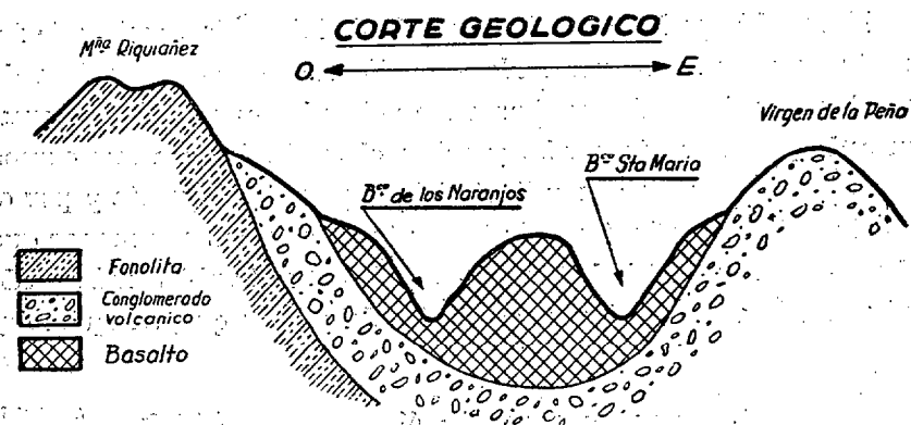
Fig. 12.—Corte geológico E. - O. de la Virgen de la Peña a Riquiáñez.
