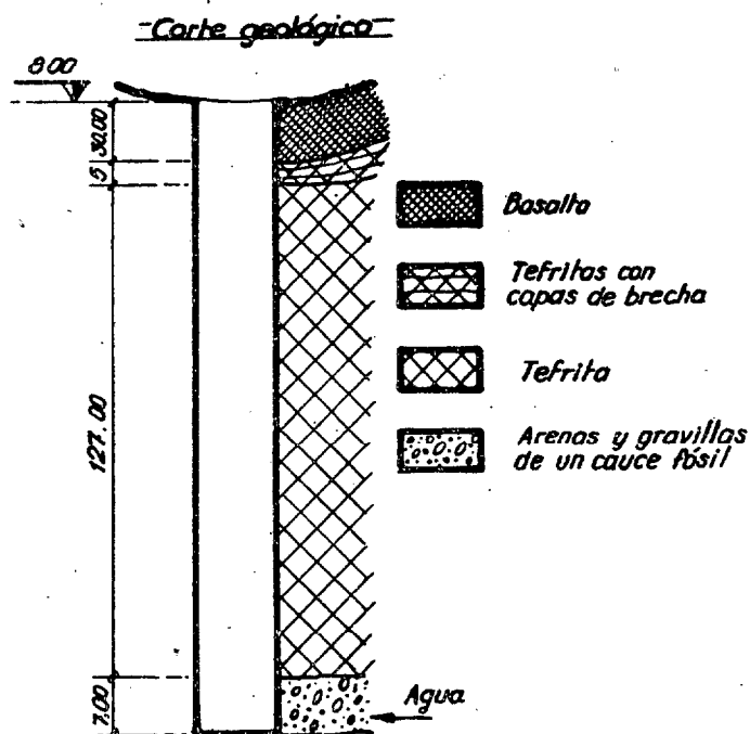
Fig. 10.—Corte geológico de un pozo abierto a la cota 800 en el Barranco de Monagas.
