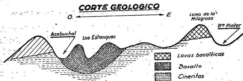
Fig. 13.—Corte geológico E. - O. cruzando el Barranco Pintor al Acebuchal.
