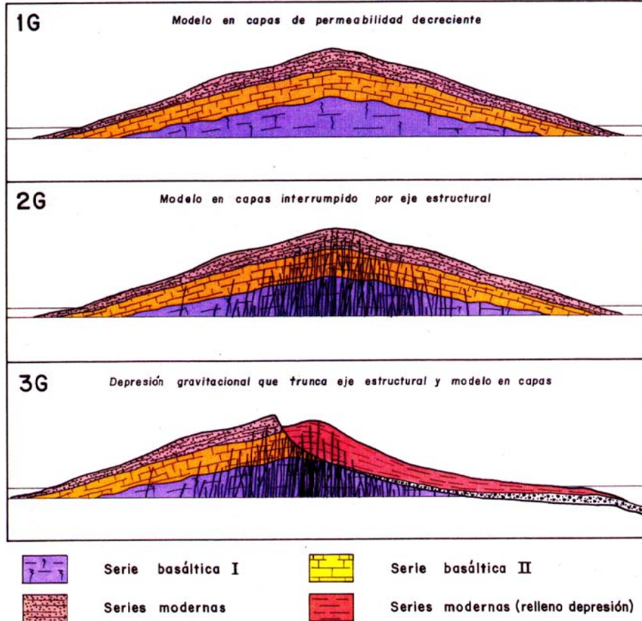
Fig. 1.- CONFIGURACION ESQUEMATICA DE LOS SUBSUELOS DE TENERIFE
