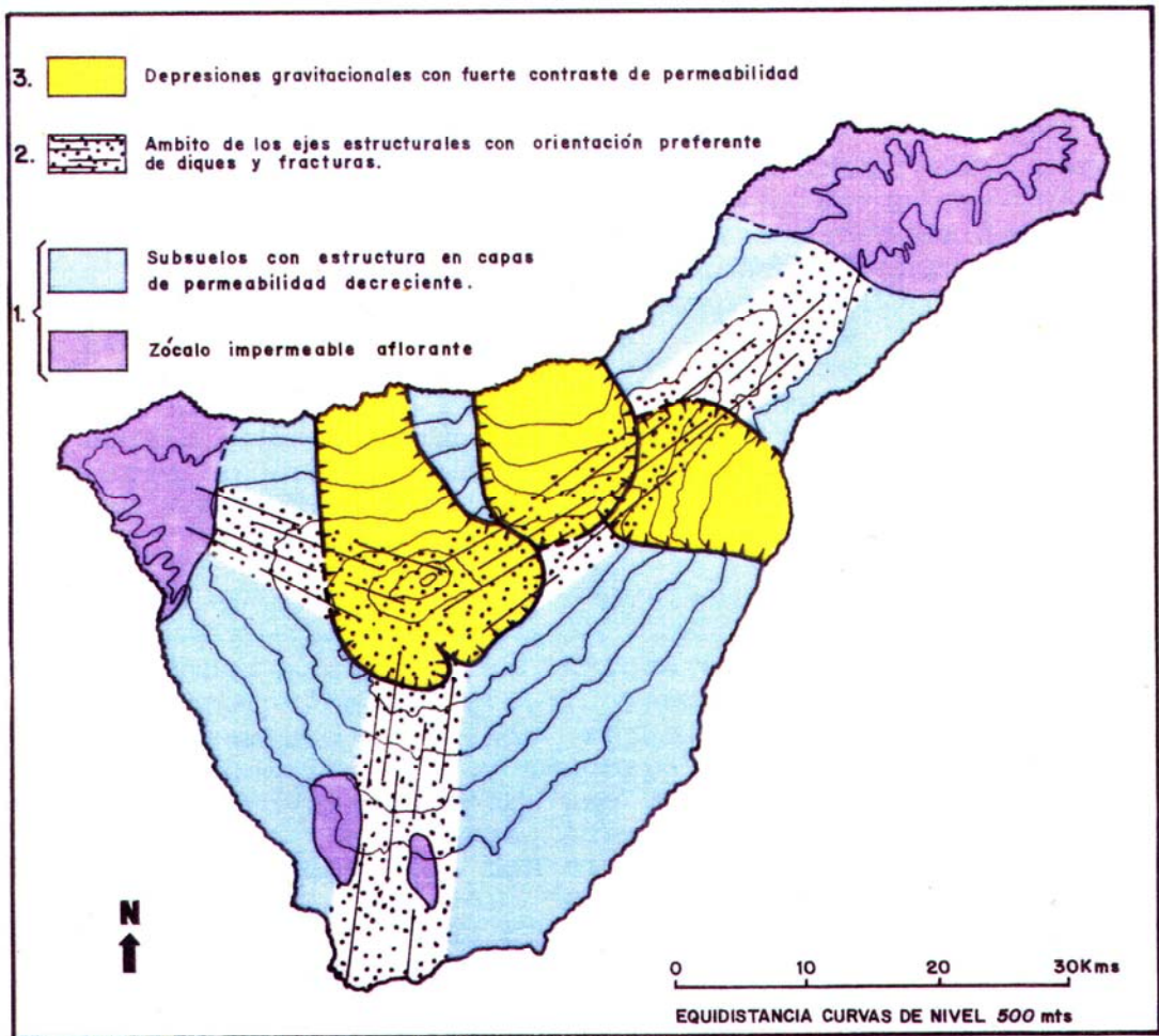
Fig.2 .- DISTRIBUCION DE LOS TIPOS DE SUBSUELOS ESQUEMATIZADOS EN LA Fig. 1 .
